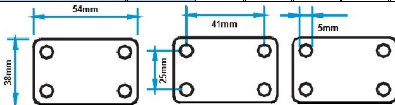
Placa fixa em formato de U com medidas do furo (41x25mm) totalmente compatíveis com placa giratória.
